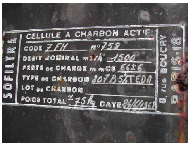
T3 / N°56 : caisson à charbon actif destiné à épurer l'air des iodes radioactifs avant insufflation dans le hangar destiné à la protection des populations lors des retombées radioactives à Rikitea (Mangareva). Débit nominal 1 500 M3/h, Date 24 juin 1968. / CRIIRAD, le 7 octobre 2005.
