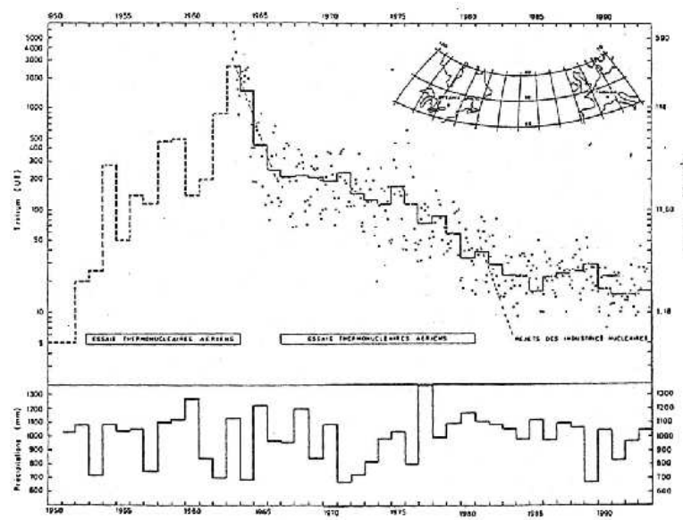
Graphique 1 : Teneurs en tritium mensuelles(•) et annuelles(-) dans les précipitations à Thonon de 1963 à 1993 ainsi que les hauteurs annuelles des précipitations [P. Olive et al, 1996].
